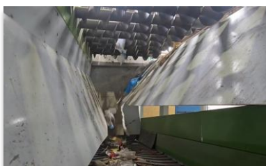
03 スクリュー羽根のピッチより小さい廃棄物はスクリーュー羽根の間から落下し下部コンベアへ排出される。
